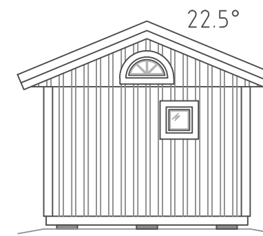
FASAD 4
