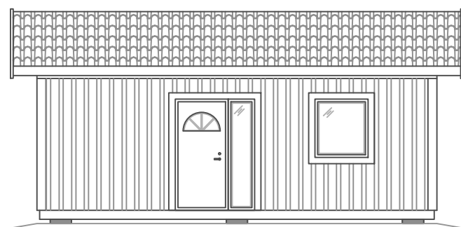
FASAD 1
